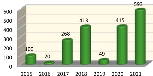
Emisja SO 2
